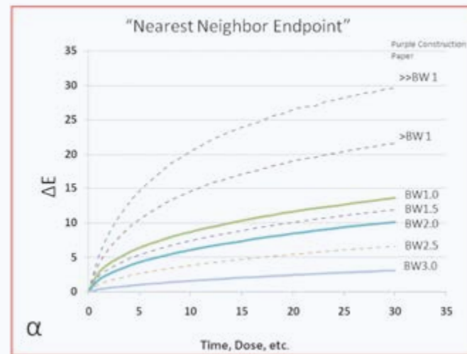
Obr. 9: Ukázka znázornění standardů BW1-3 a jejich vypočítaných ekvivalentů BWE (> BW1, BW1,5 a BW2,5). Křivka pro hodnotu >> BW1 byla změněna na nevybledlém růžovém papíru pro technické výkresy. [16] Celková barevná změna \Delta E byla vypočítána dle rovnice (2).
